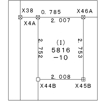
拡大図 S=1:100
